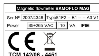
Rys. Etykieta konwertera
