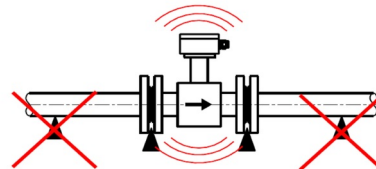
Rys. 12 - Ryzyko wibracji
