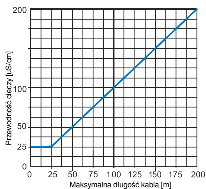
Rys.23 - Maksymalna długość kabla, a przewodność
