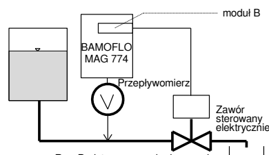
Rys. Podstawowa opcja dozowania
