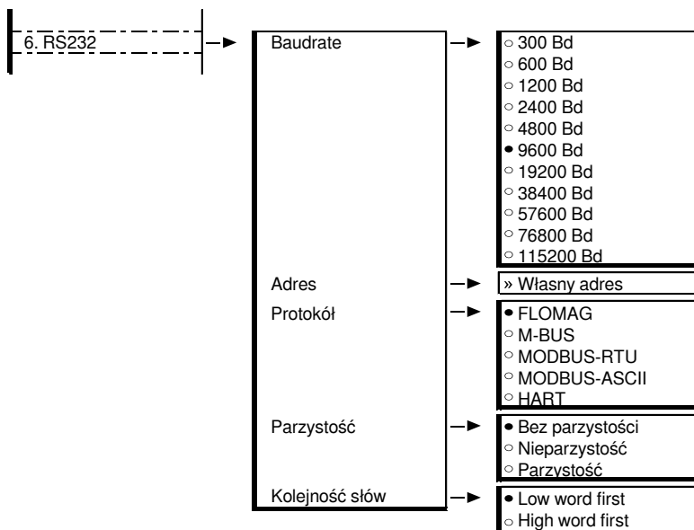
Rys. Menu modułu komunikacyjnego
