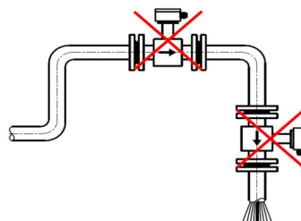
Rys. 10 - Ryzyko zapowietrzenia
