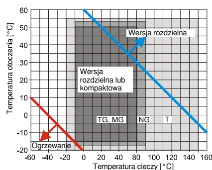
Rys.24 - Wybór wersji w zależności od temperatury
