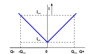
Rys. Wyjście IQI
