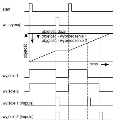
Rys. Dozowanie w trakcie
