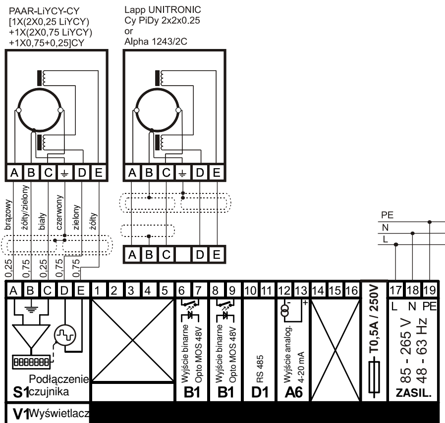
Rys.22 - Podłączenie wersji rozdzielnej
