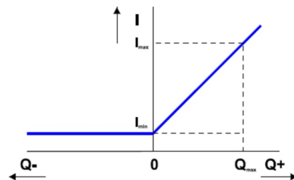
Rys. 0 ... Q wyjście
