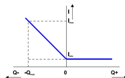
Rys. 0 ... -Q wyjście
