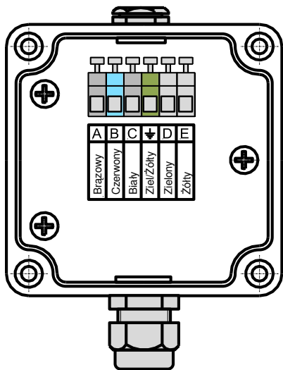
Rys. 21 - Skrzynka przyłączeniowa czujnika
