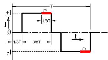
Rys.2 - Kształt impulsu wzbudzającego
