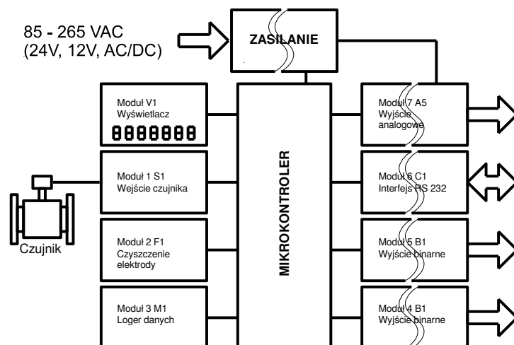
Rys.19 - Schemat blokowy przepływomierza
