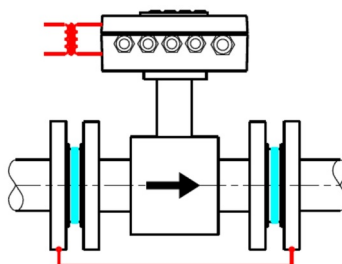
Rys.18 - Ochrona katodowa
