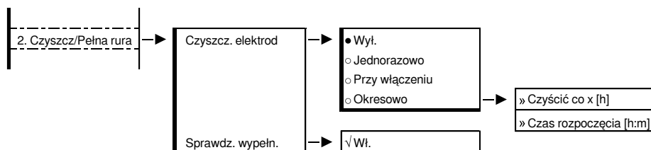
Rys. Menu modułu F3
