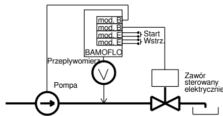
Rys. Złożona opcja dozowania
