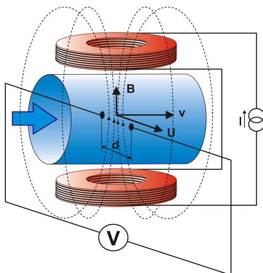
Rys.1 - Zasada pomiaru
