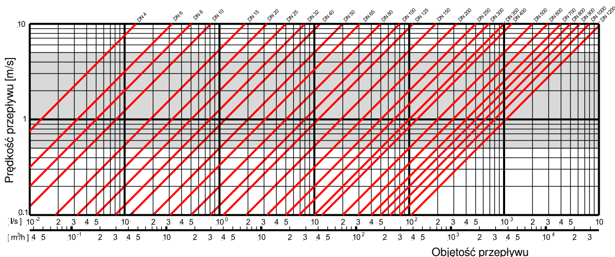
Schemat prawidłowego doboru przepływomierza
