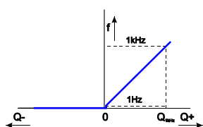
Rys. Częstotliwość Q+
