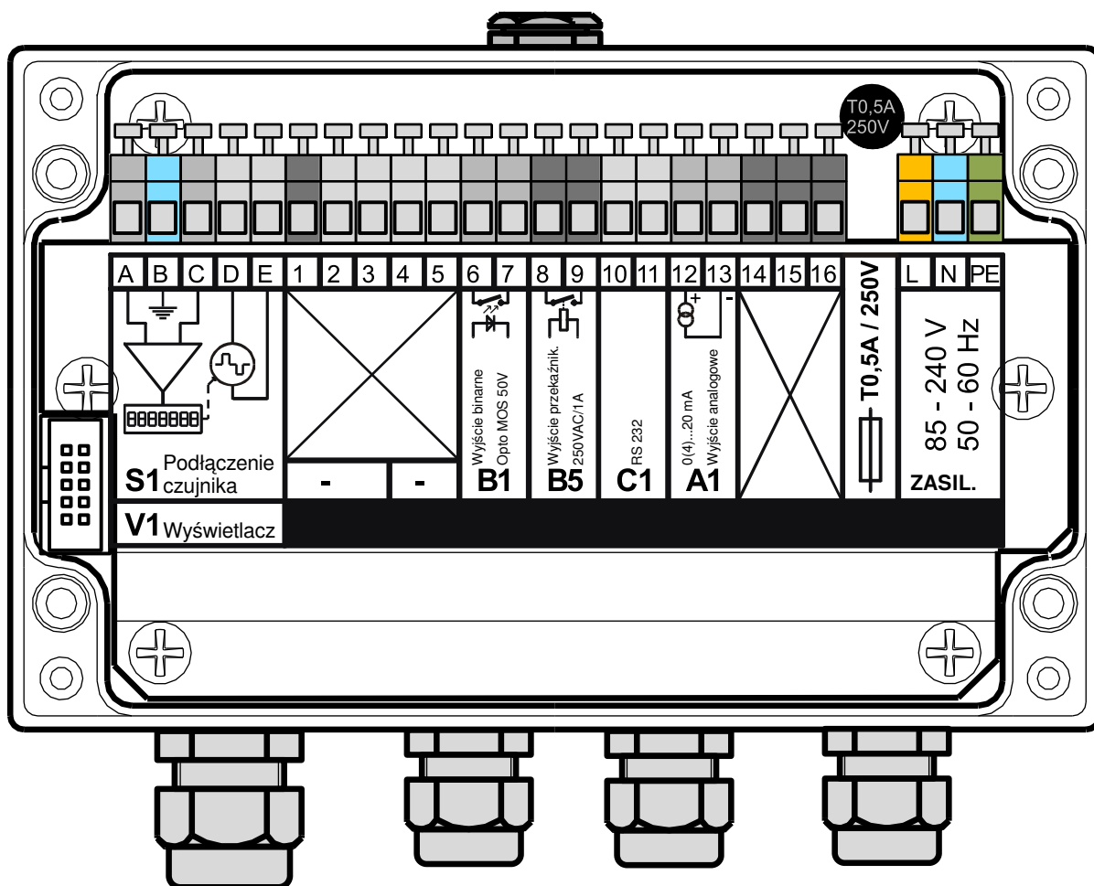
Rys.20 - Lokalizacja zacisków konwertera
