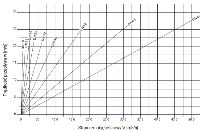
Wykres - Ilość powietrza (SV 91)
