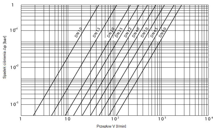
Wykres - Przepływ - spadek ciśnienia (SV 95)
